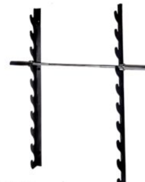
Настенный кронштейн для 10 грифов, горизонтальное хранение (комплект)
